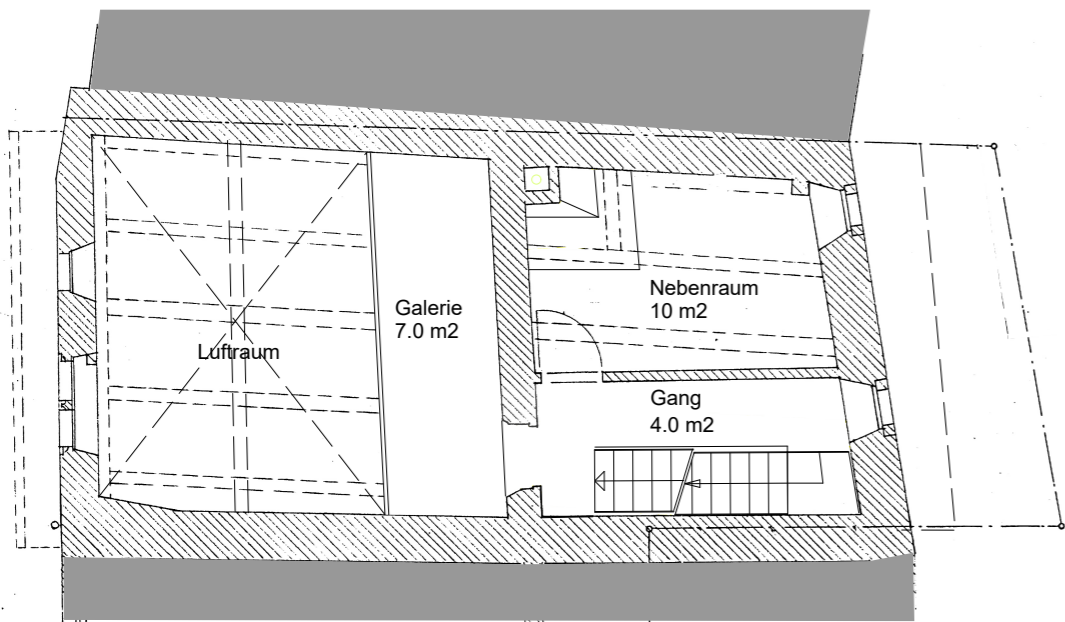
GRUNDRISS ZWISCHENGESCHOSS
