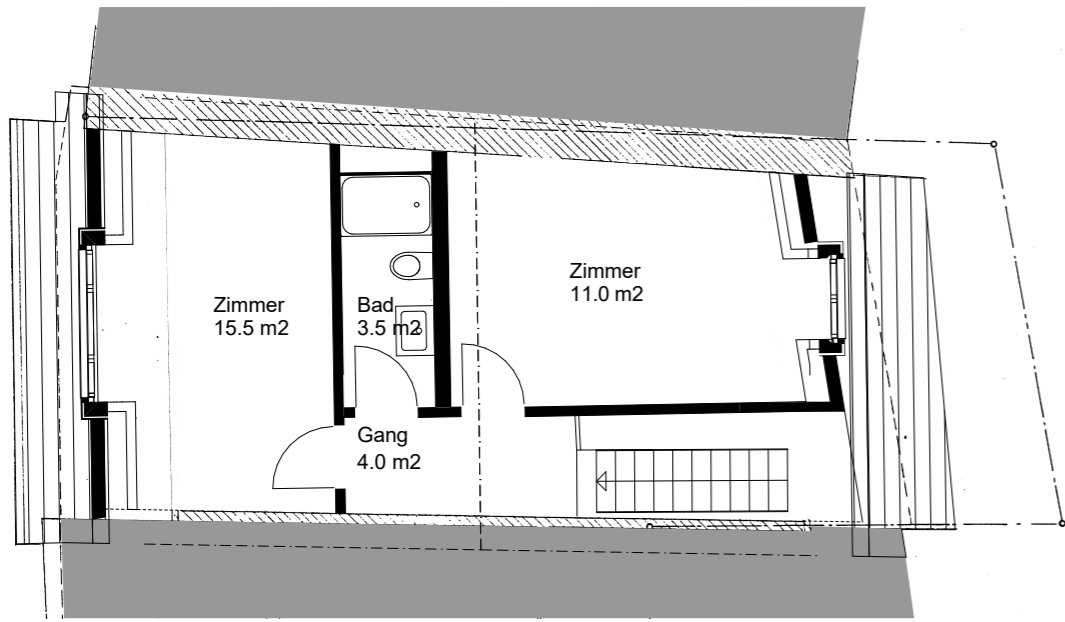
GRUNDRISS DACHGESCHOSS
