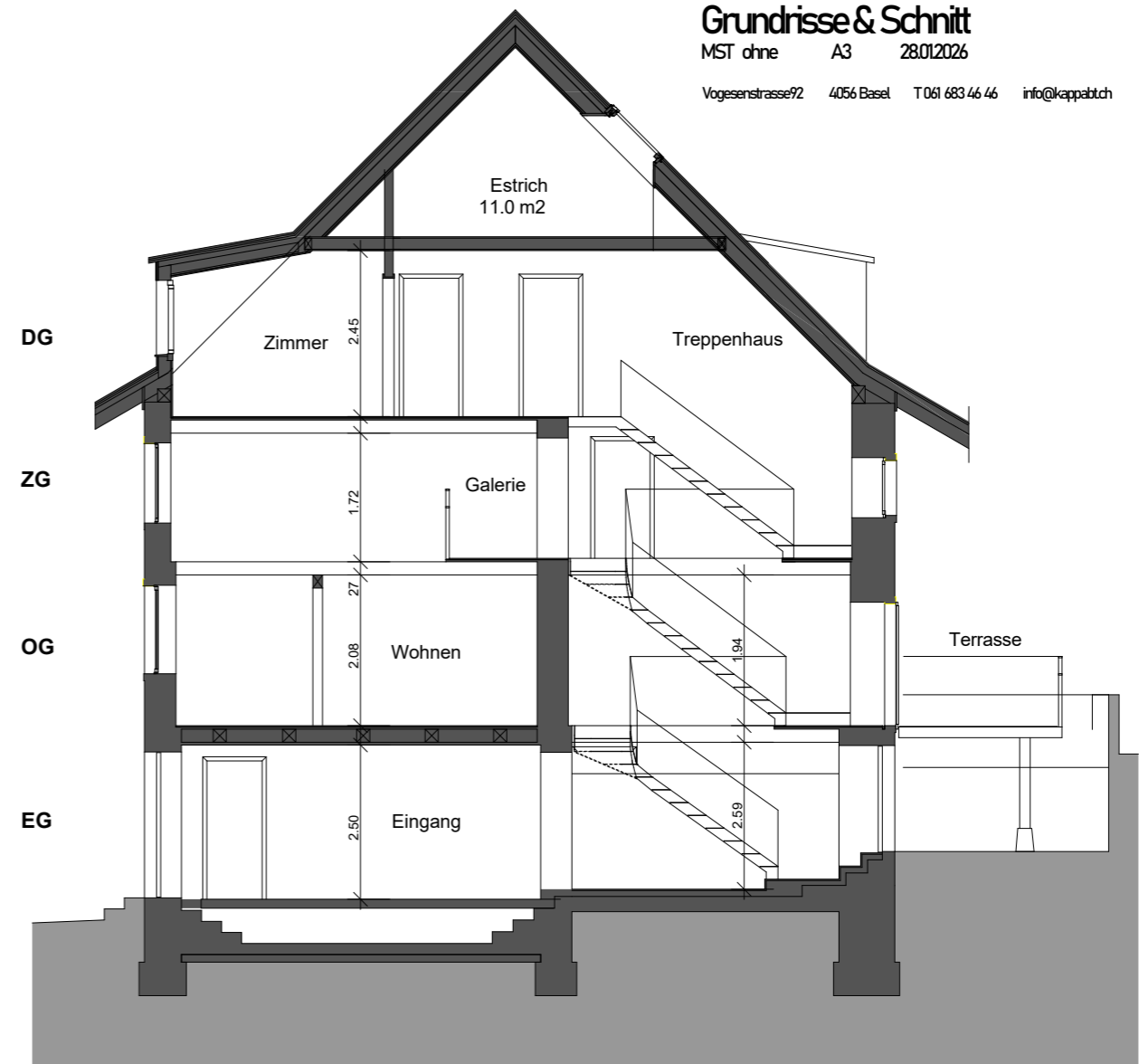
QUERSCHNITT
