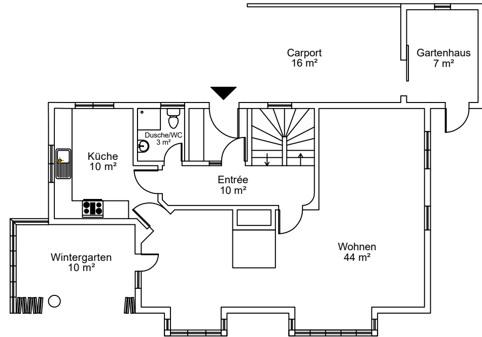
ERDGESCHOSS
