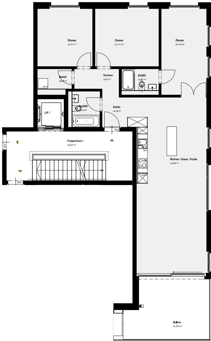
Grundriss Wohnung
