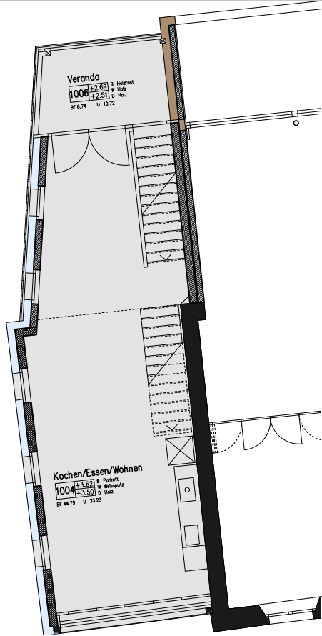
1. Obergeschoss
