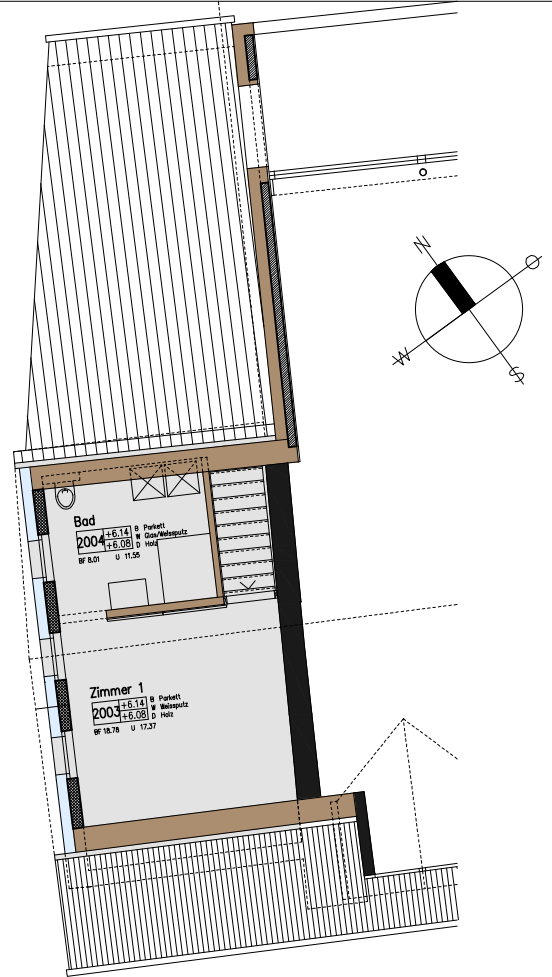
1. Dachgeschoss
