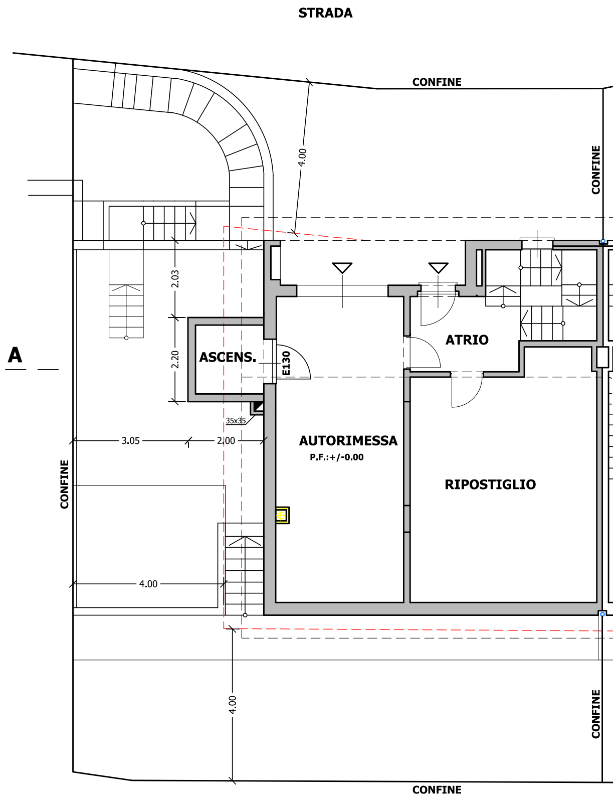
PIANTA PIANO ENTRATA
