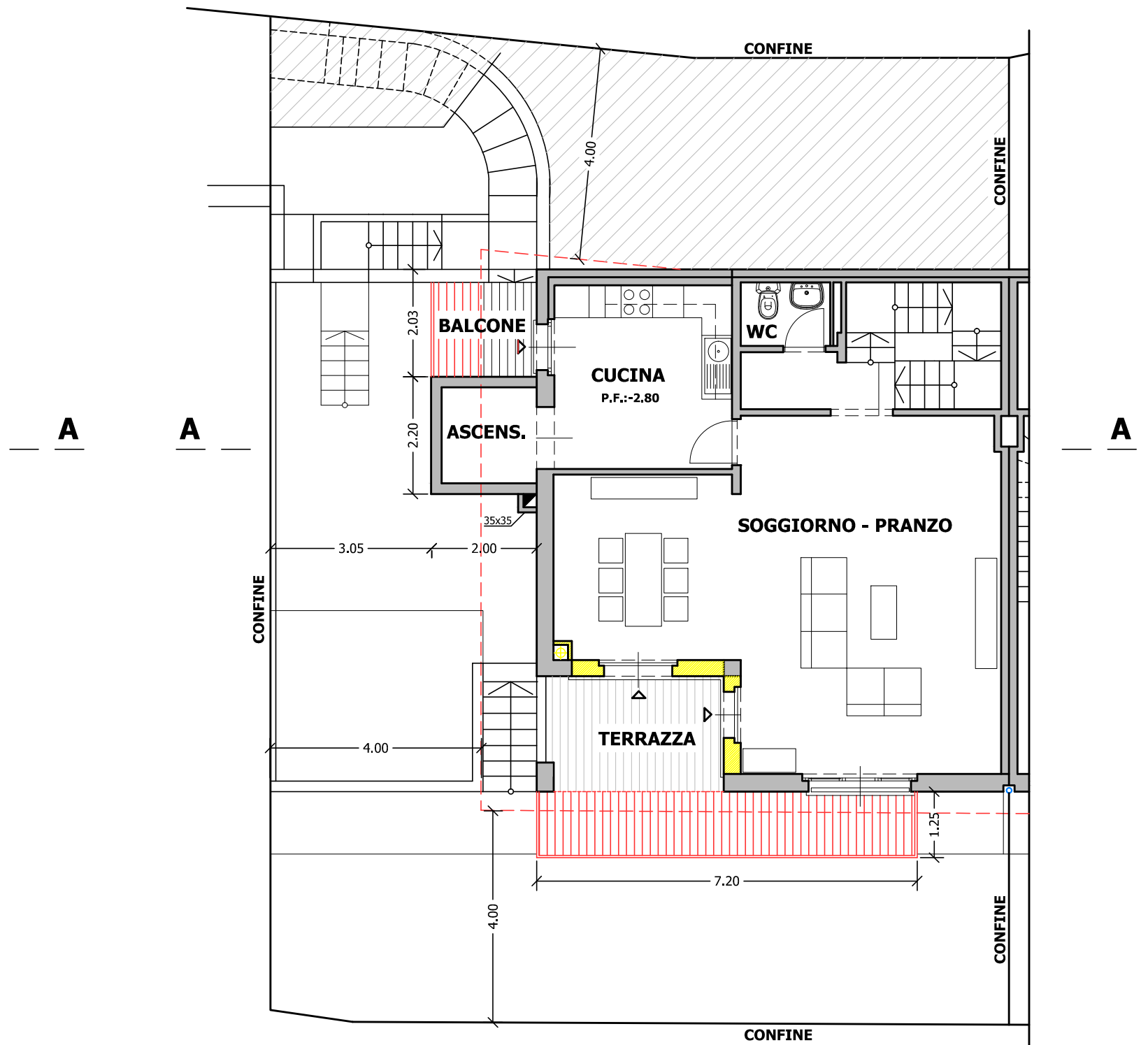
PIANTA PIANO GIORNO
