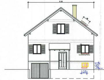
Nordfassade 1 : 100
