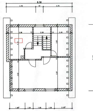
Grundriss Obergeschoss 1 : 100
