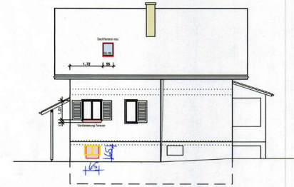
Westfassade 1 : 100
