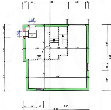
Grundriss Untergeschoss 1 : 100
