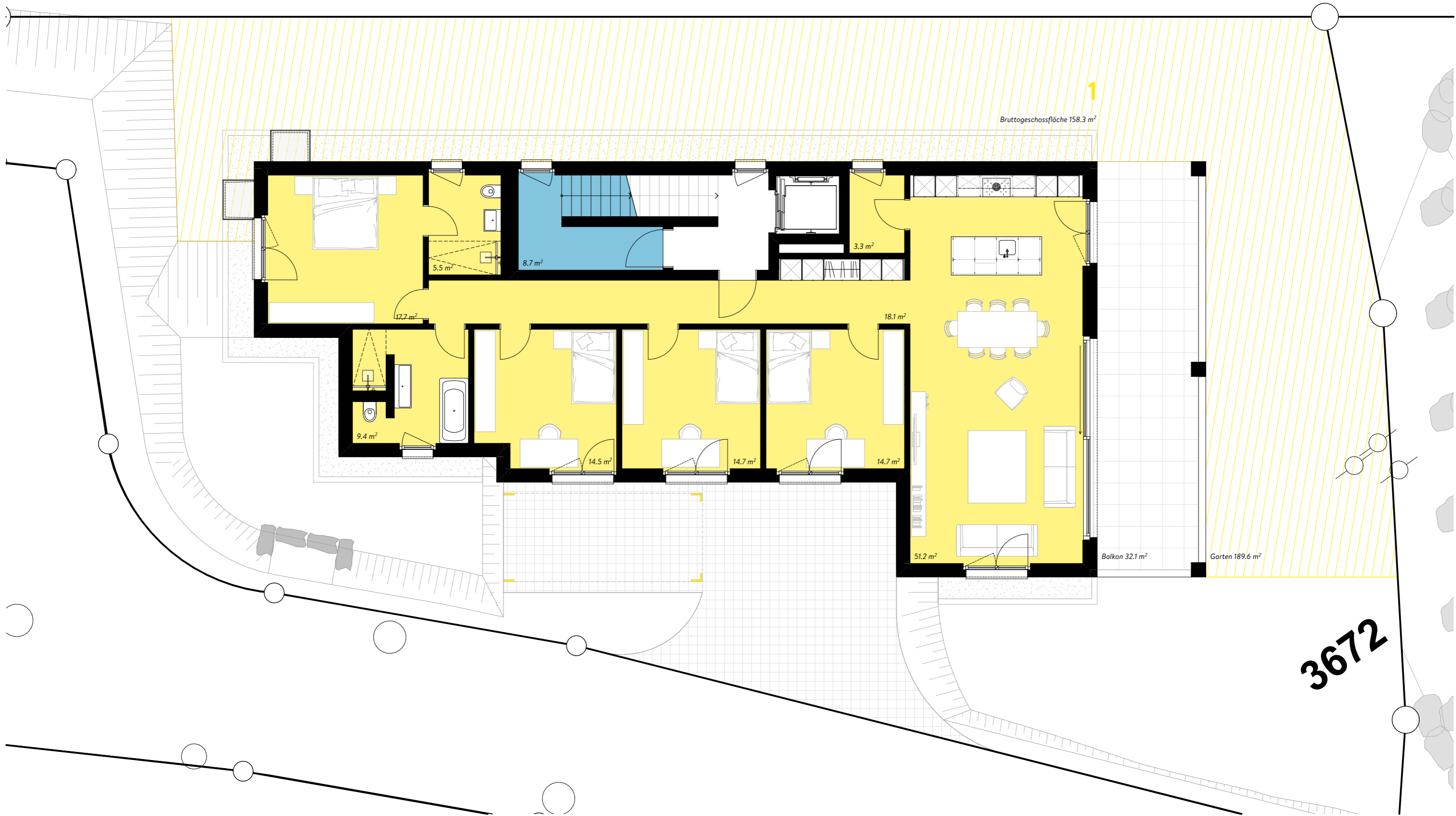
Seengen Erdgeschoss Wohnung Nr.1 1:100
