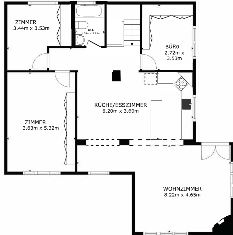
STOCKWERK 2
