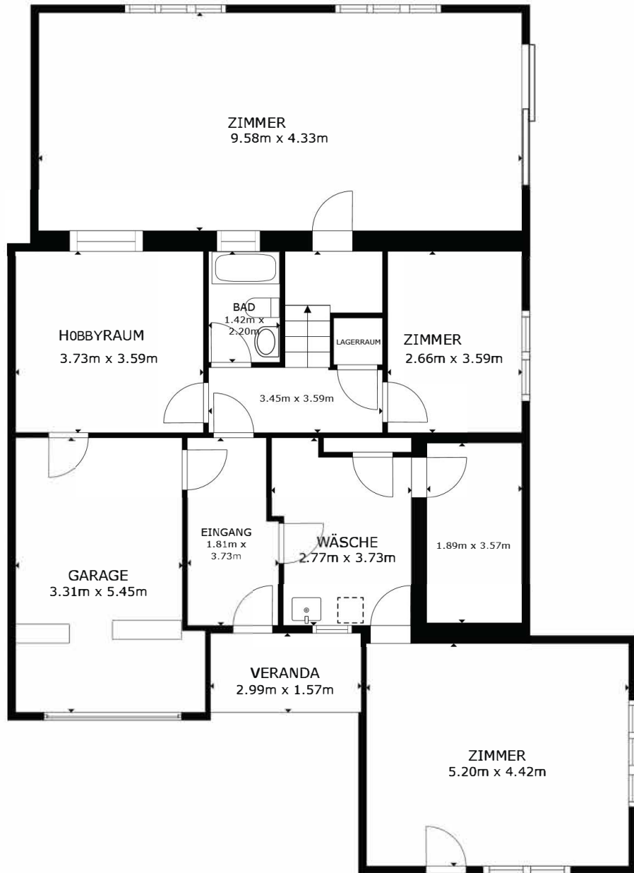
STOCKWERK 1
