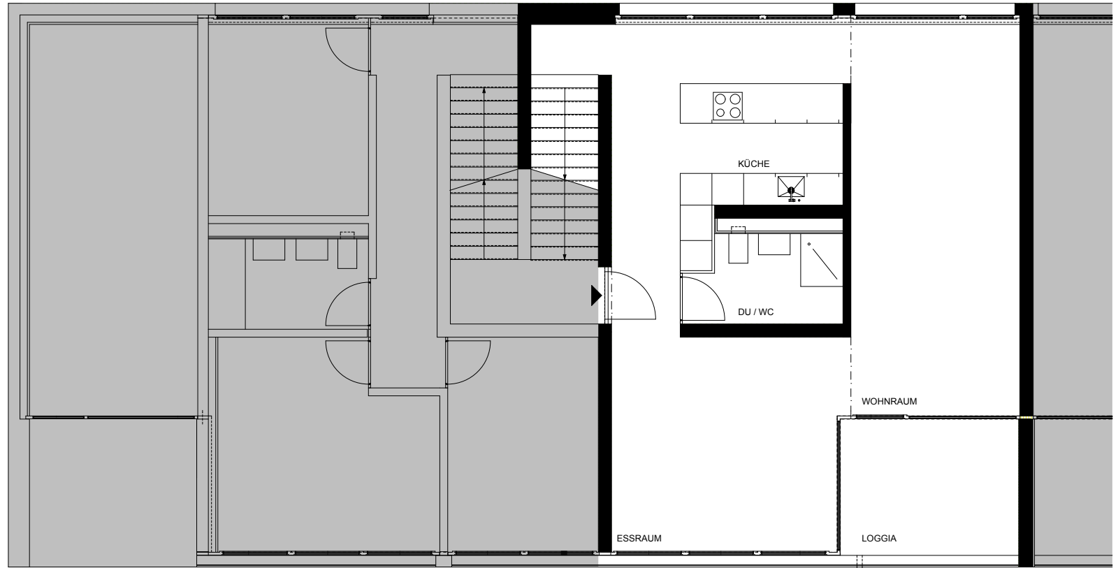
MEHRFAMILIENHAUS UNTERE KRÄZERN HAUS 2 WOHNUNG 3 2.OG
