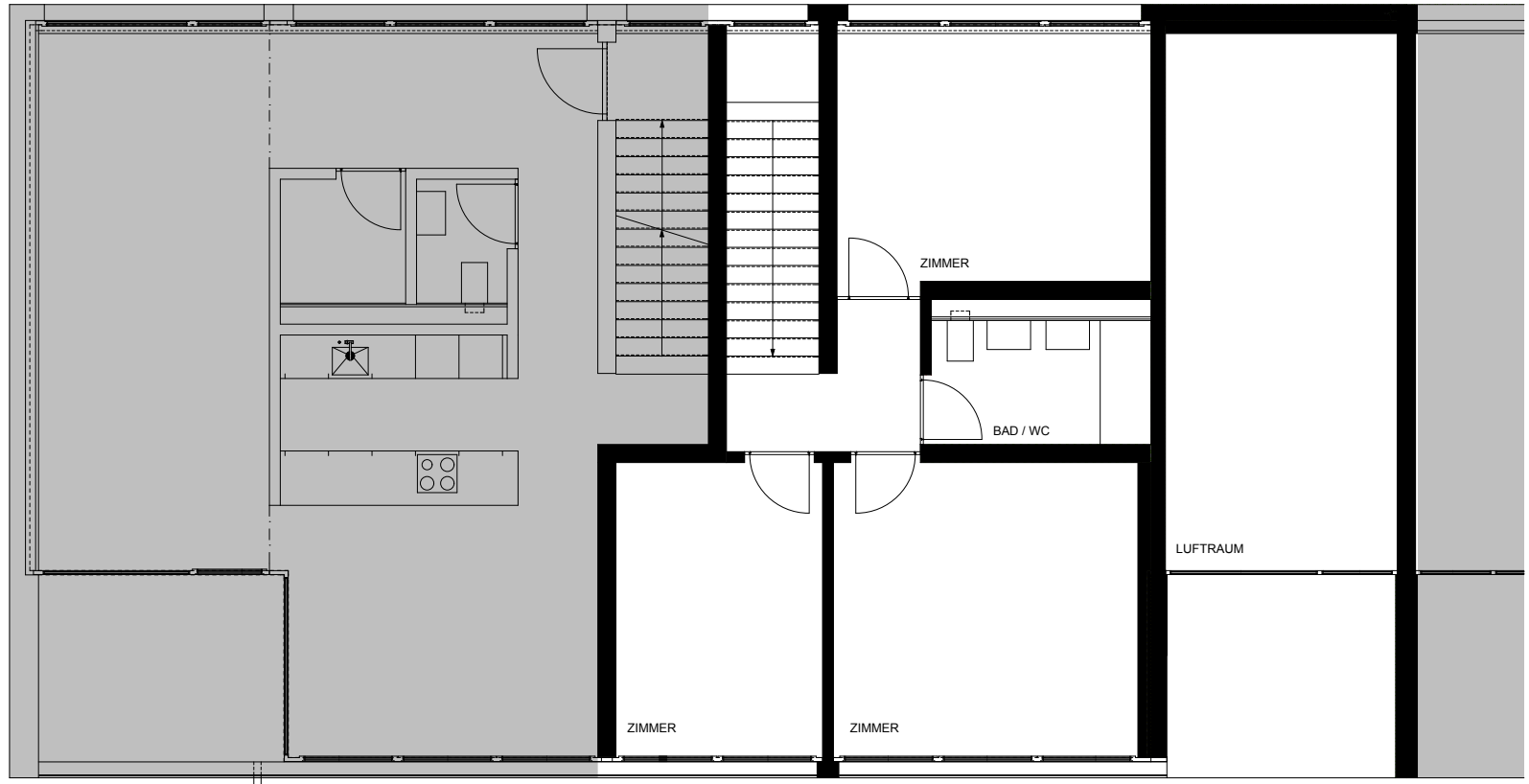
MEHRFAMILIENHAUS UNTERE KRÄZERN HAUS 2 WOHNUNG 3 3.OG
