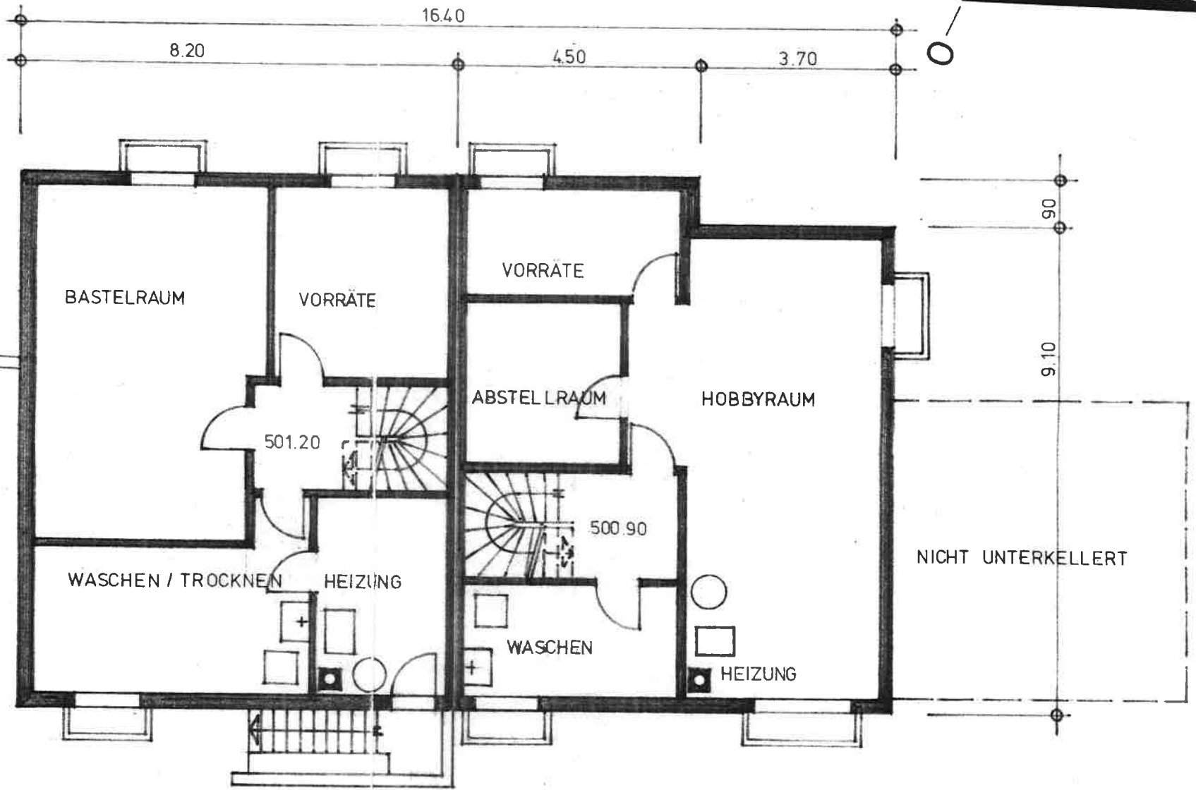
GRUNDRISS UNTERGESCHOSS
