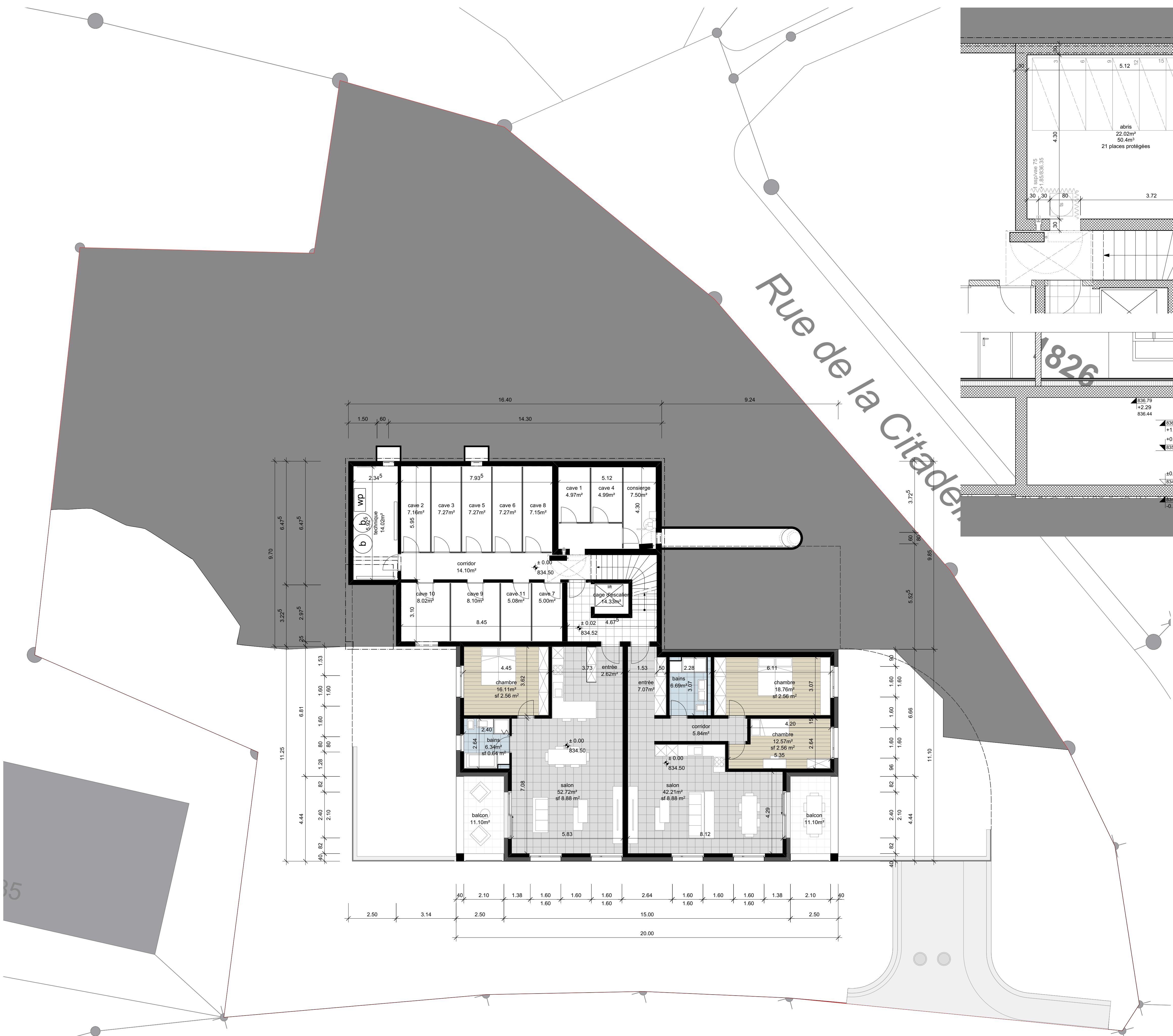
abris de la protection civile - planimétrie 1:50
