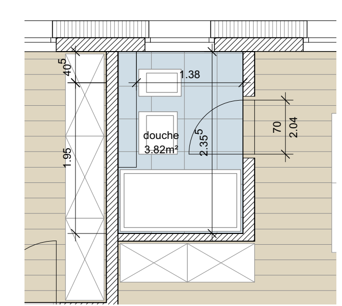
détail 1:50 - douche - appartements 3, 6 et 9 n'ais pas selon la norme sia 500
