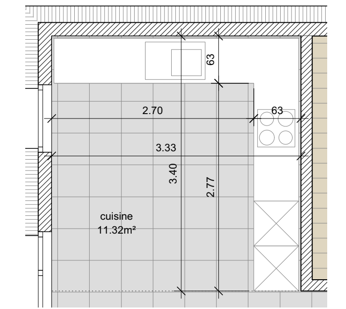
détail 1:50 - cuisine - appartements 3, 6 et 9
