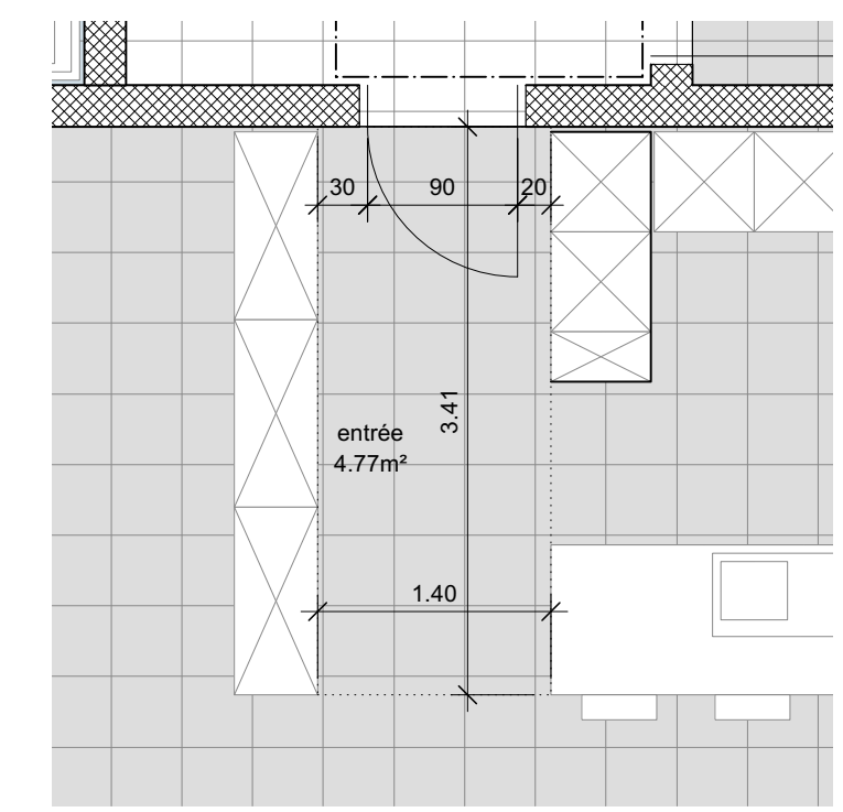
détail 1:50 - entrée - appartement 10
