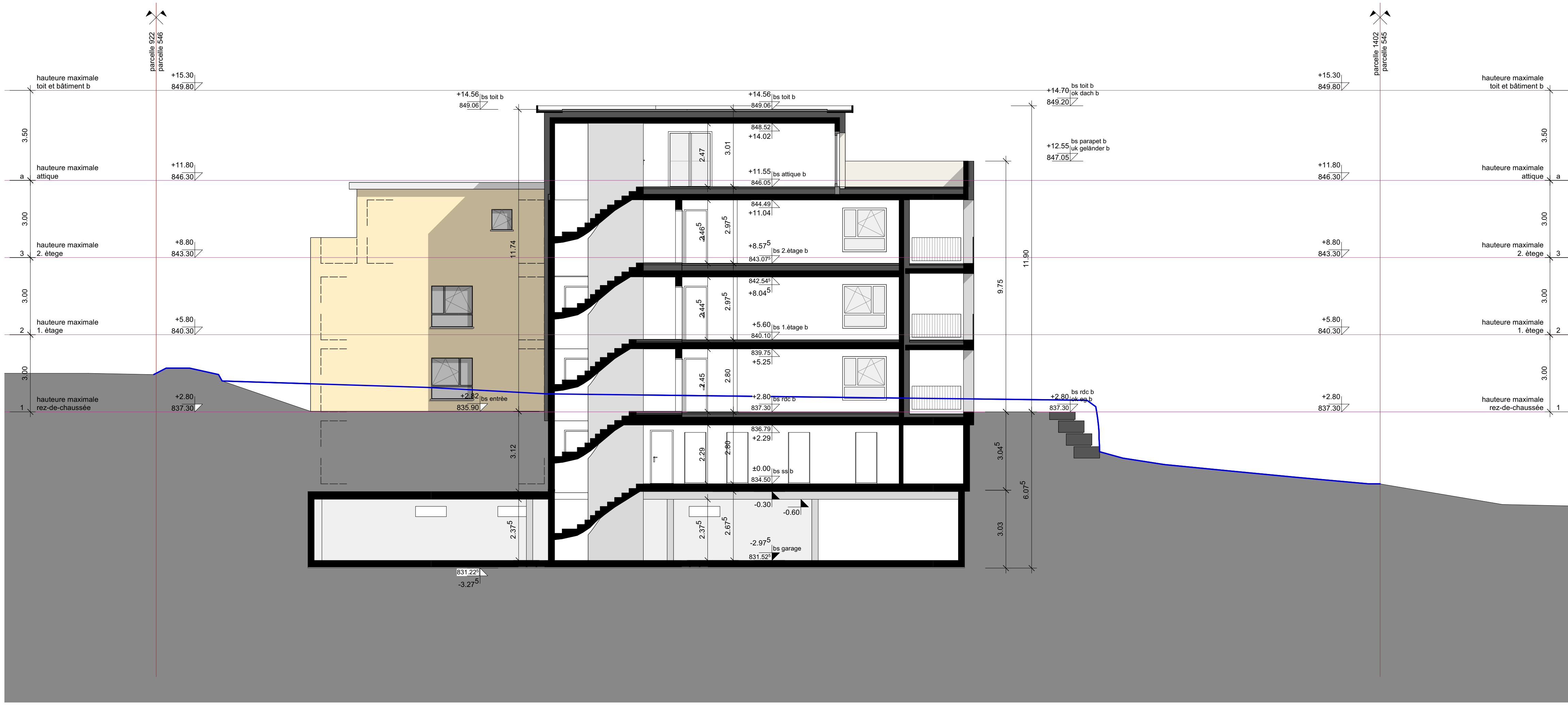
coupe a-a
