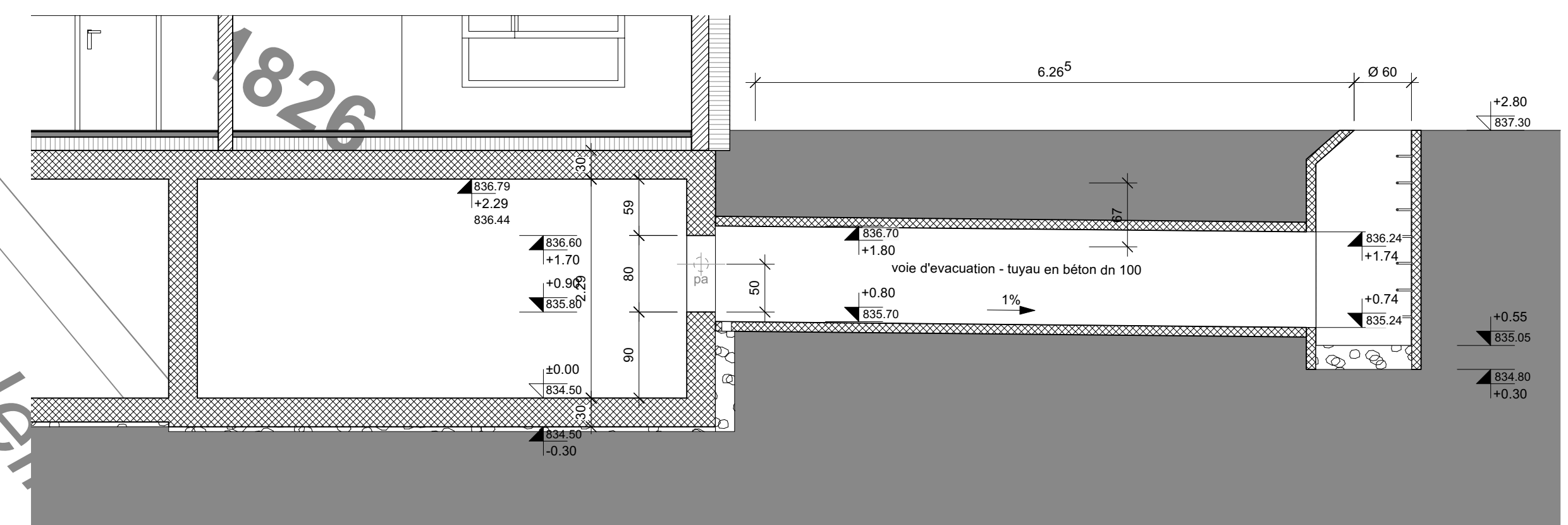
abris de la protection civile - coupe 1:50
