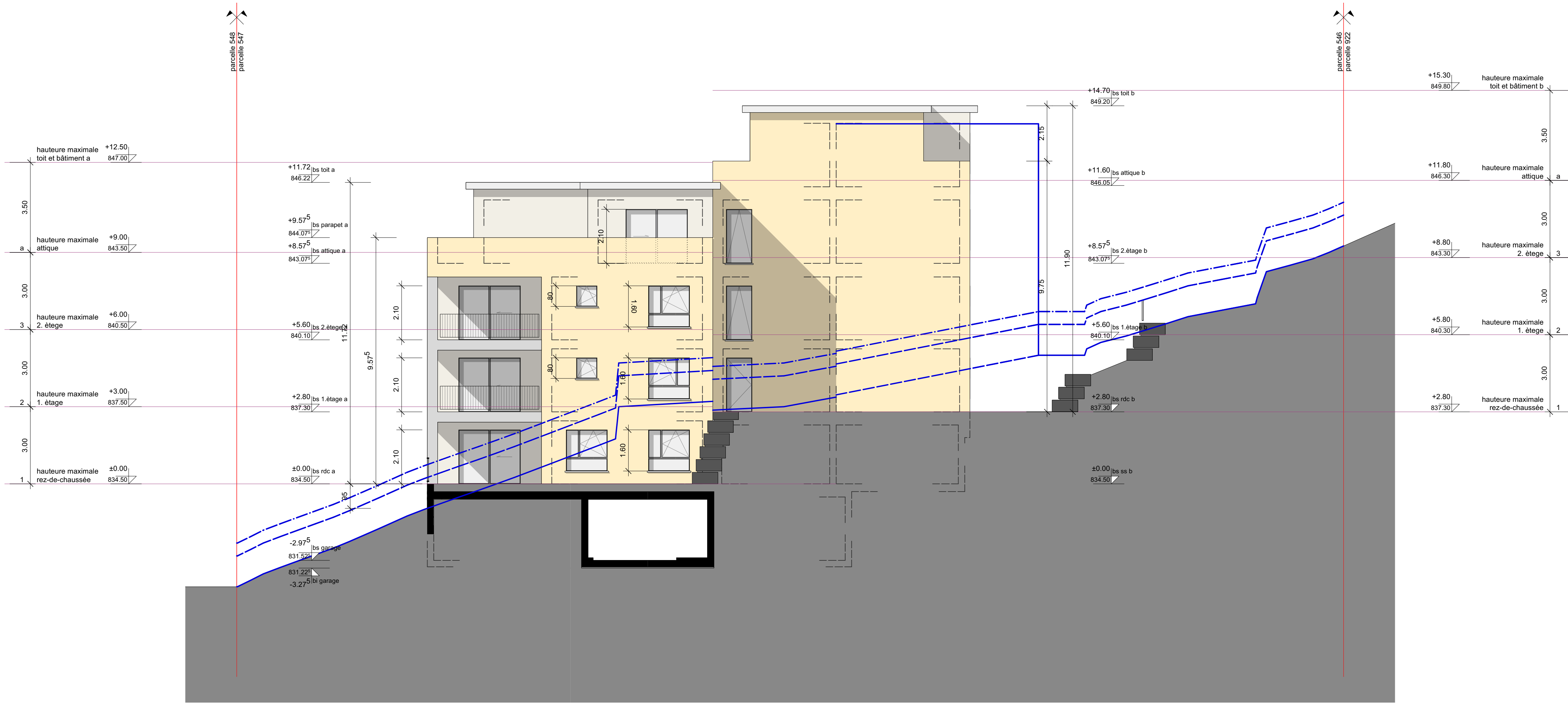
vue est
