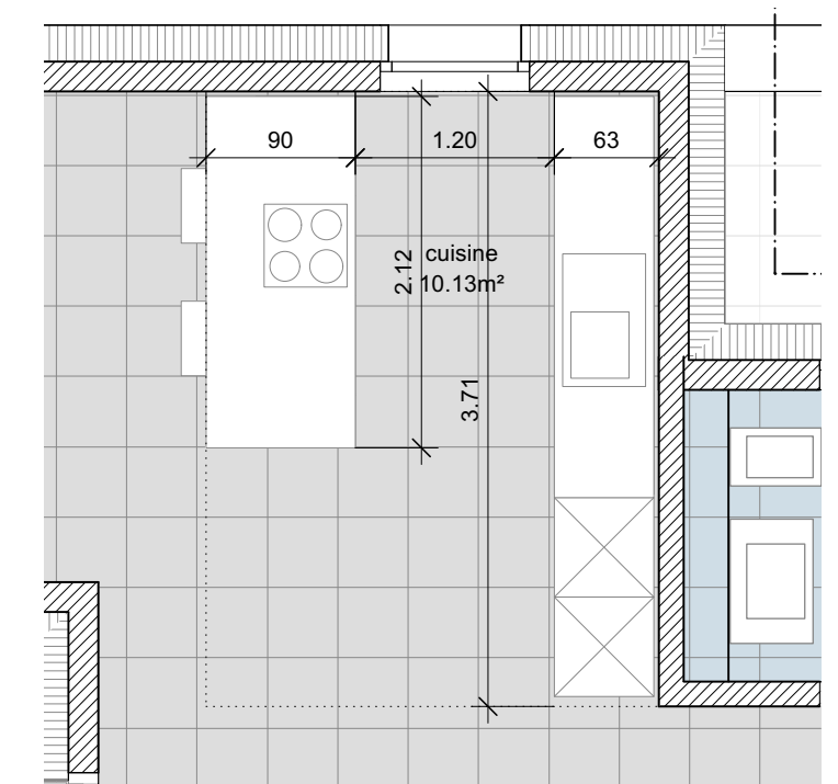
détail 1:50 - cuisine - appartement 11
