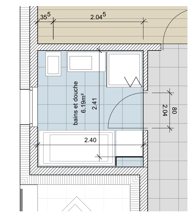
détail 1:50 - salle de bains - appartements 1, 4 et 7 selon la norme sia 500
