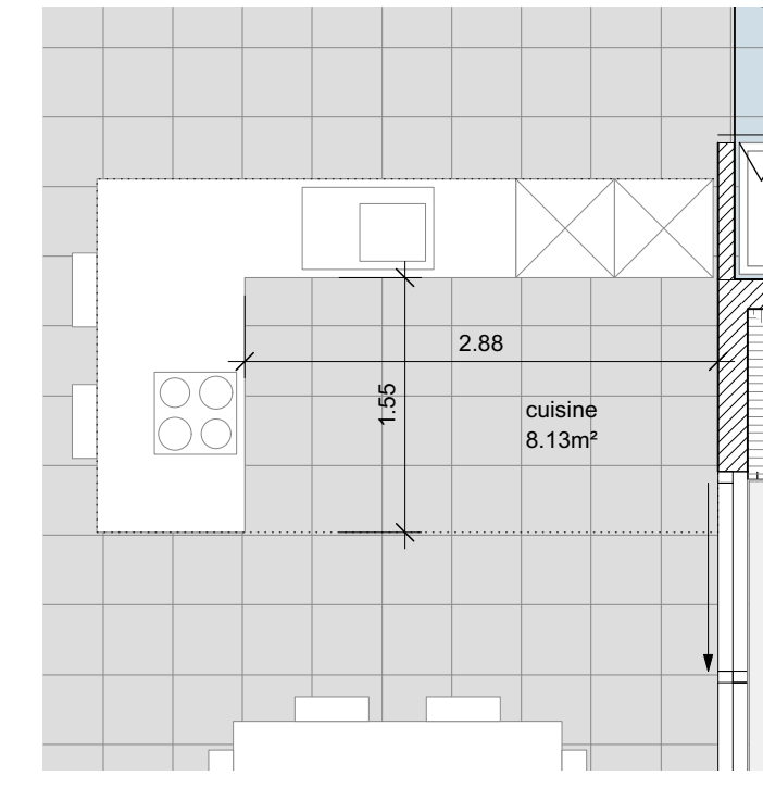
détail 1:50 - cuisine - appartements 2, 5 et 8
