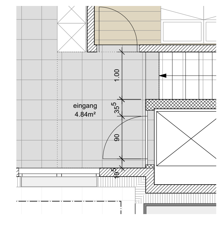
détail 1:50 - entrée - appartement 11
