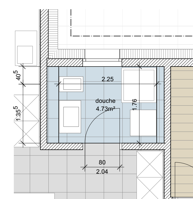
détail 1:50 - douche - appartement 11 selon la norme sia 500
