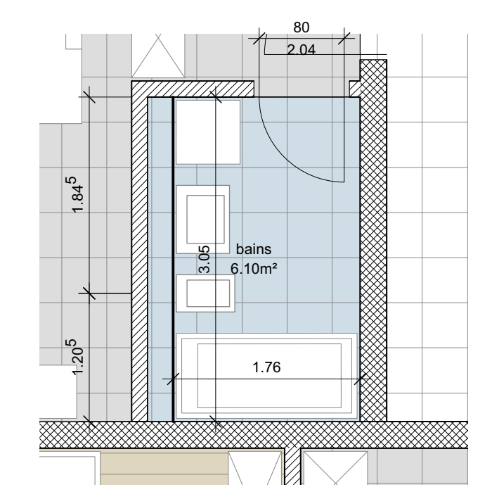
détail 1:50 - salle de bains - appartements 3, 6 et 9 selon la norme sia 500
