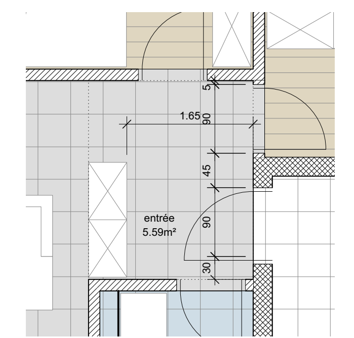
détail 1:50 - entrée - appartements 3, 6 et 9
