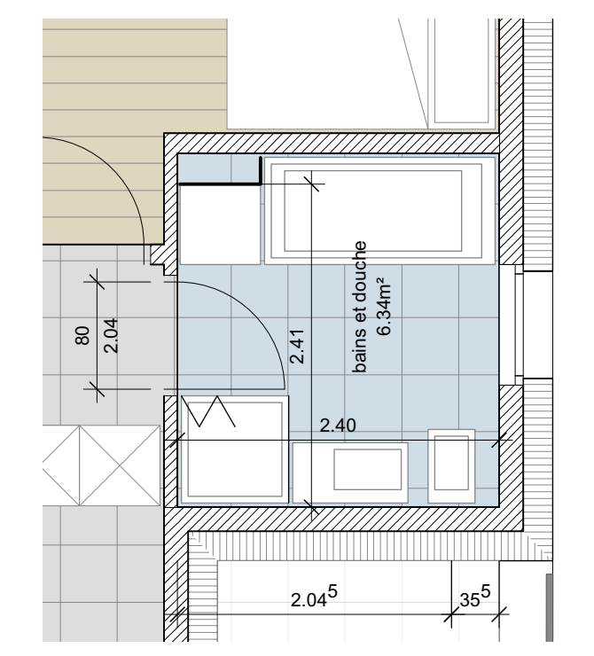
détail 1:50 - salle de bains - appartements 5 et 8 selon la norme sia 500
