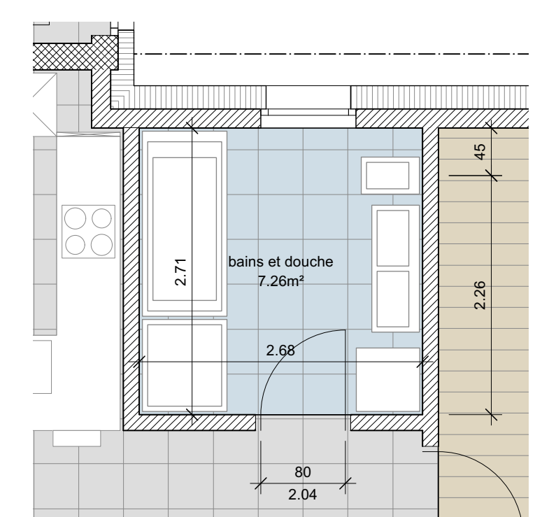
détail 1:50 - salle de bains - appartement 10 selon la norme sia 500
