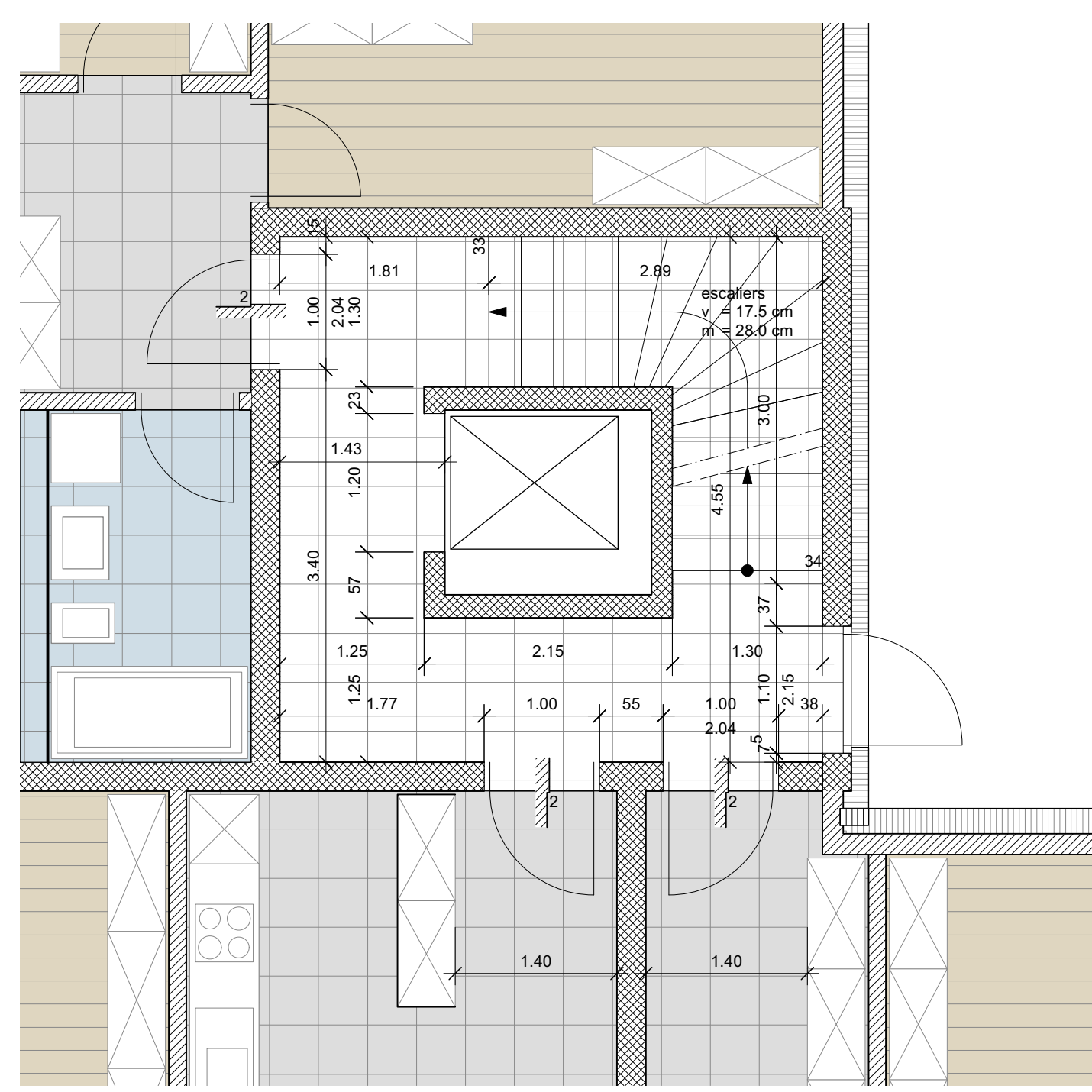
cage d'escalier detail 1:50
