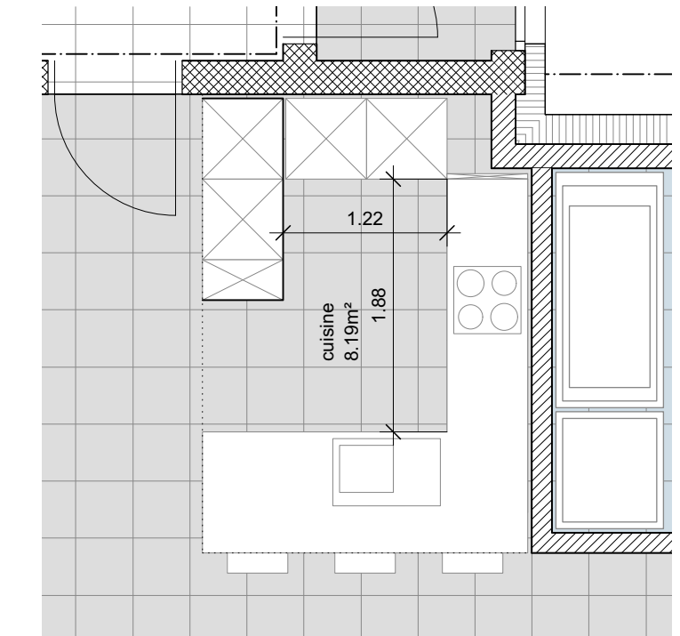
détail 1:50 - cuisine - appartement 10
