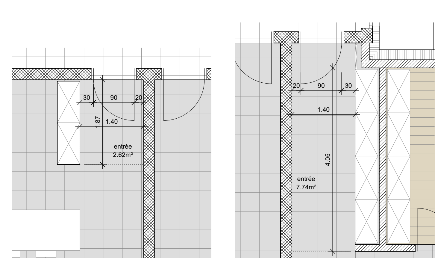
détail 1:50 - entrée - appartements 1, 4 et 7
