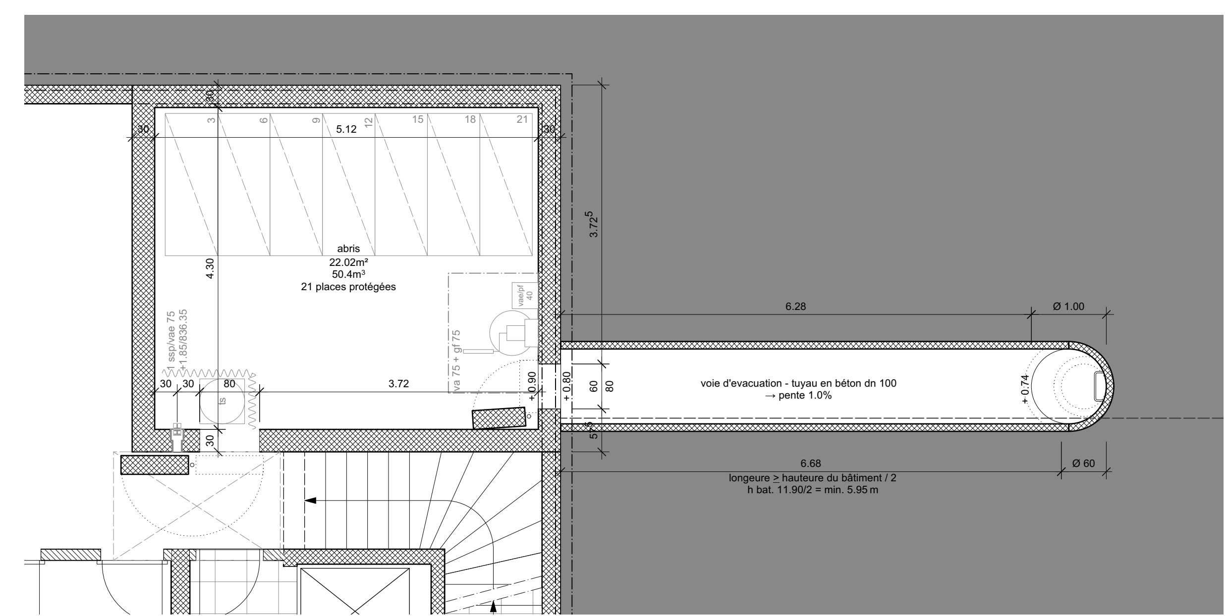
abris de la protection civile - planimétrie 1:50
