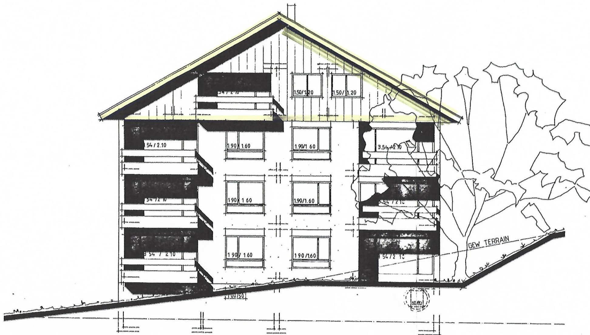
Ost-Fassade 1 : 100
