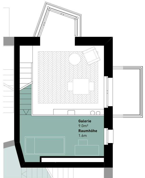
Grundriss Galerie
