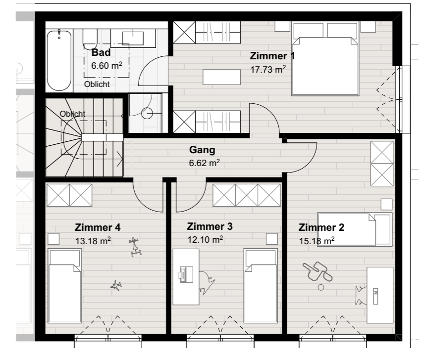
Obergeschoss 1:100
