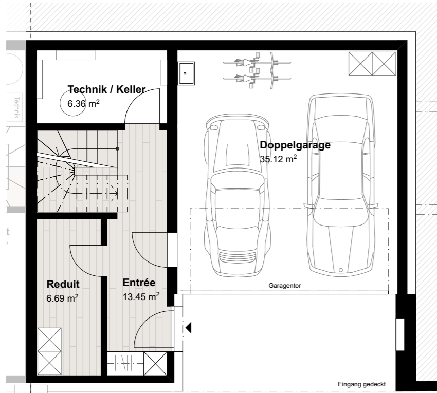
Untergeschoss 1:100
