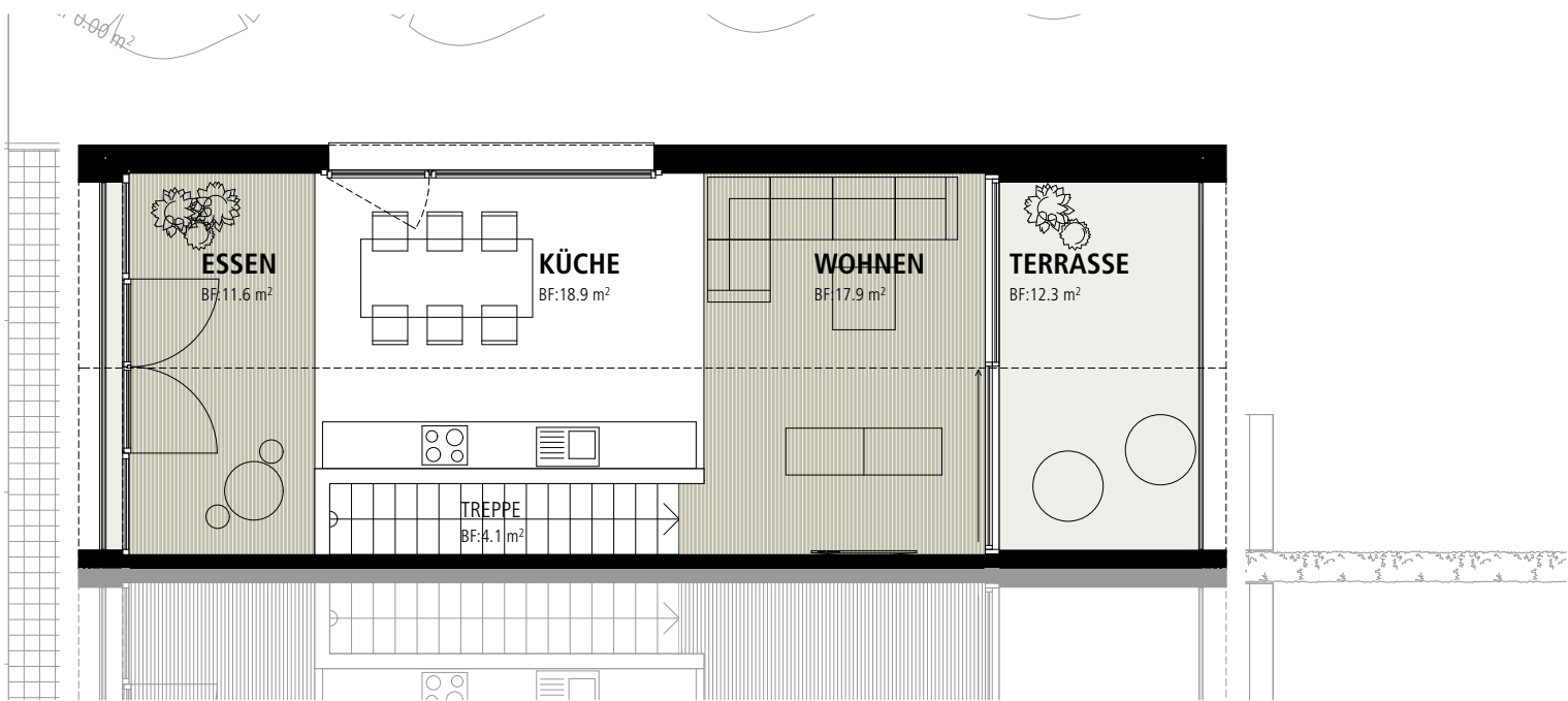
OBERGESCHOSS
