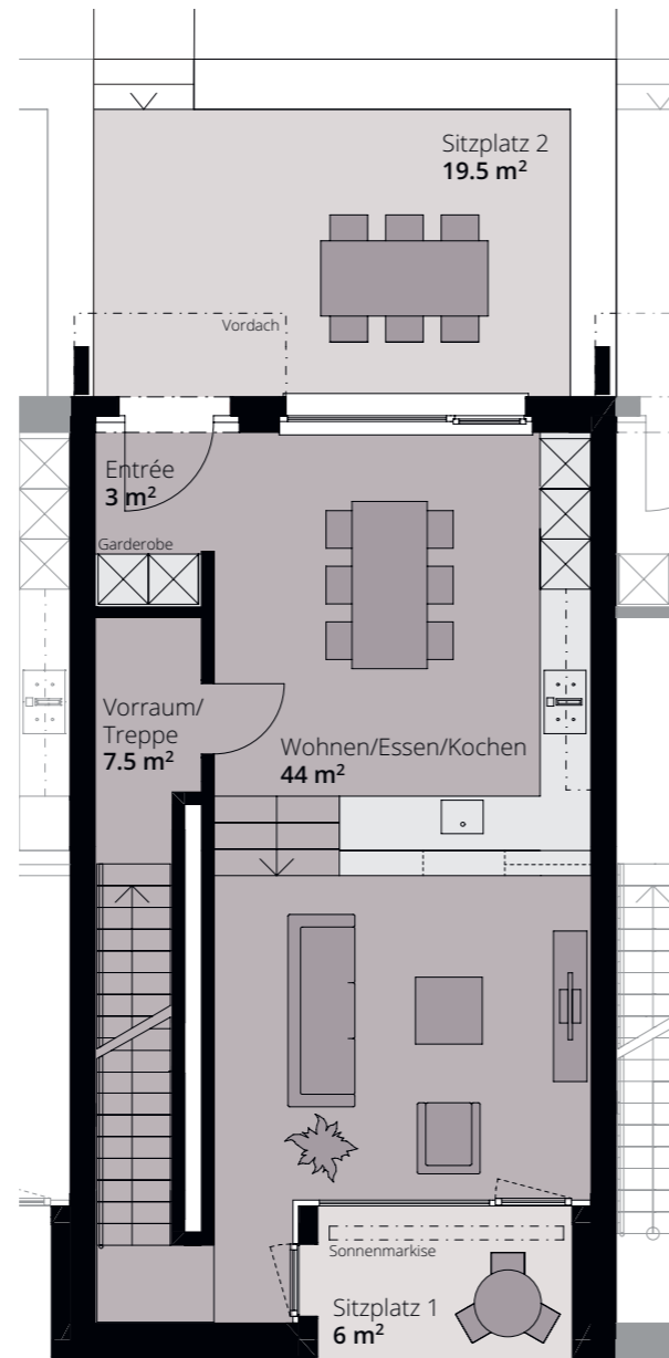
Erdgeschoss
