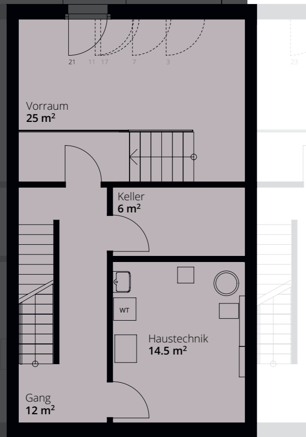
Untergeschoss
