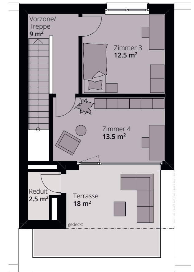
2. Obergeschoss
