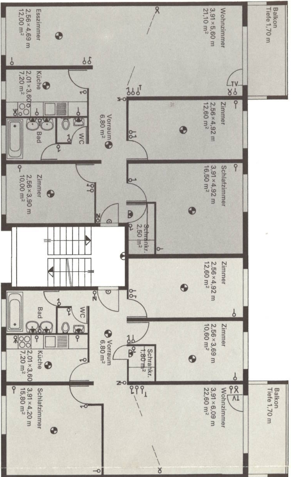
5 -Zimmer-Wohnung links
