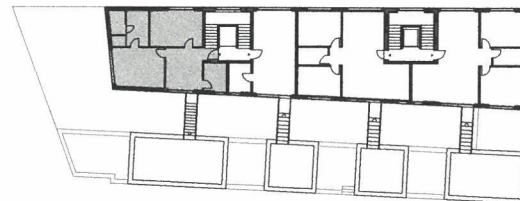
2. Obergeschoss Grundriss 1:500 Ⓞ
