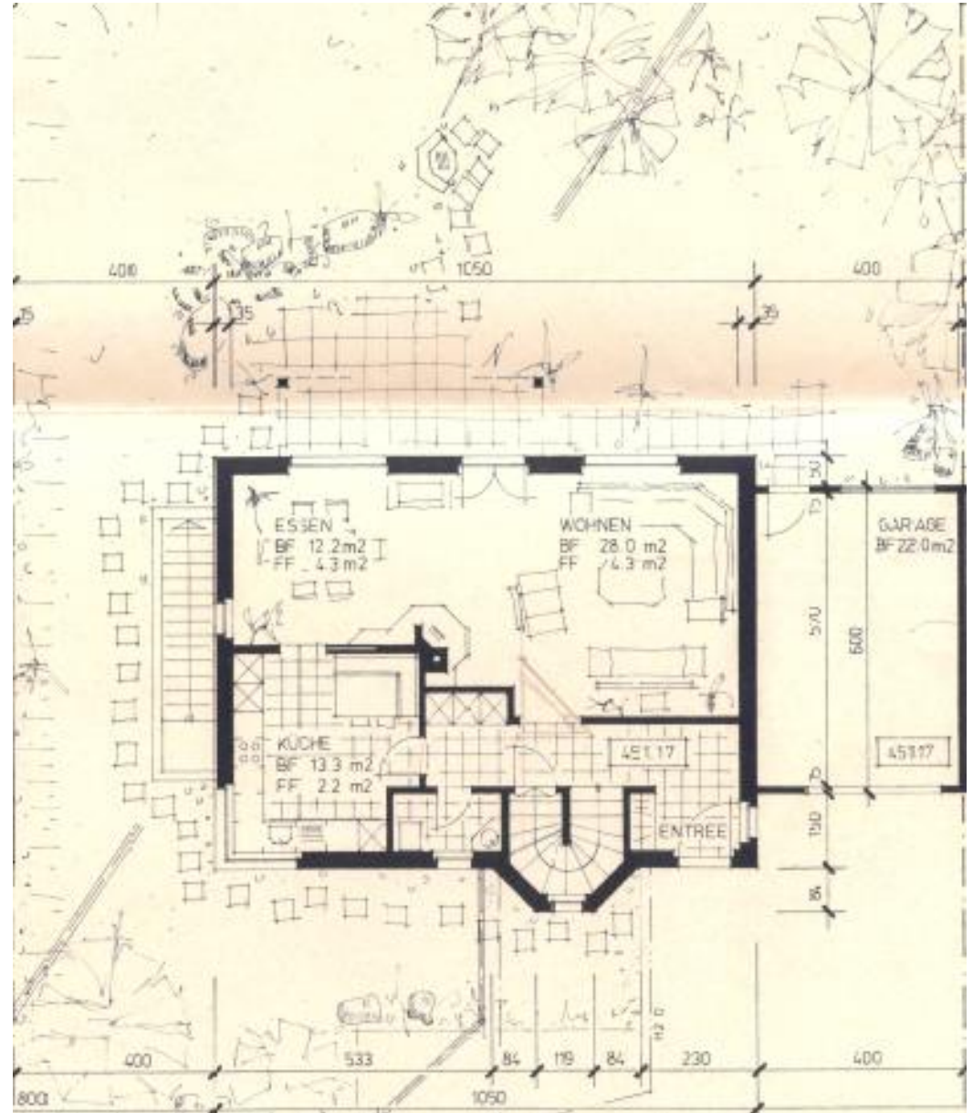
Erdgeschoss
