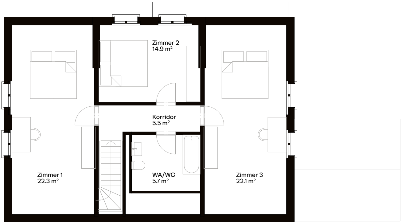
A302 – Dachgeschoss
