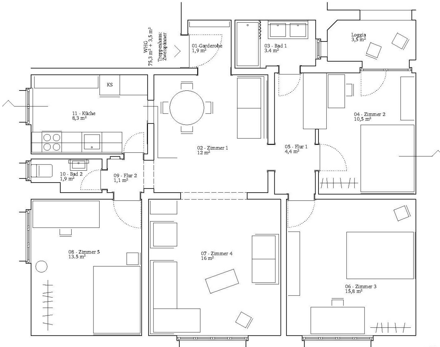
Abb. 03: Möblierter Grundriss
