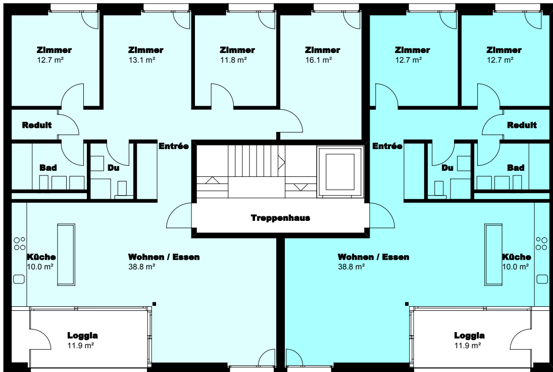
Grundriss M. 1:150
