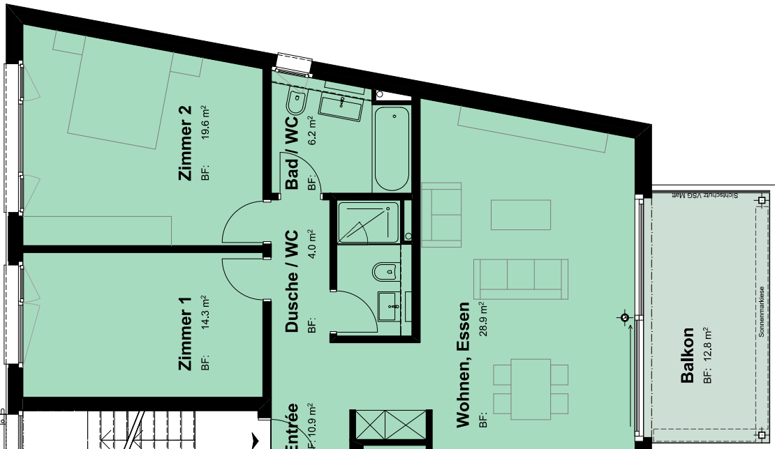
Wohnung 1.2 - NWF 97,3m 2 + 12,8m 2 Balkon
